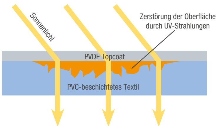
Einfluss von UV-Strahlung auf die Grenzschicht zwischen Lack und PVC-Oberfläche bei einem normalen ROWAFLON® Lacksystem.
